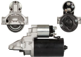
LES0309 12V / 2.0kW 12 Teeth
