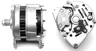
LEA0056 14V / 65A
