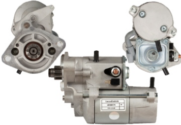
LES0274 12V / 2.0kW 9 Teeth
