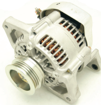
LEA0564 14V / 110A
